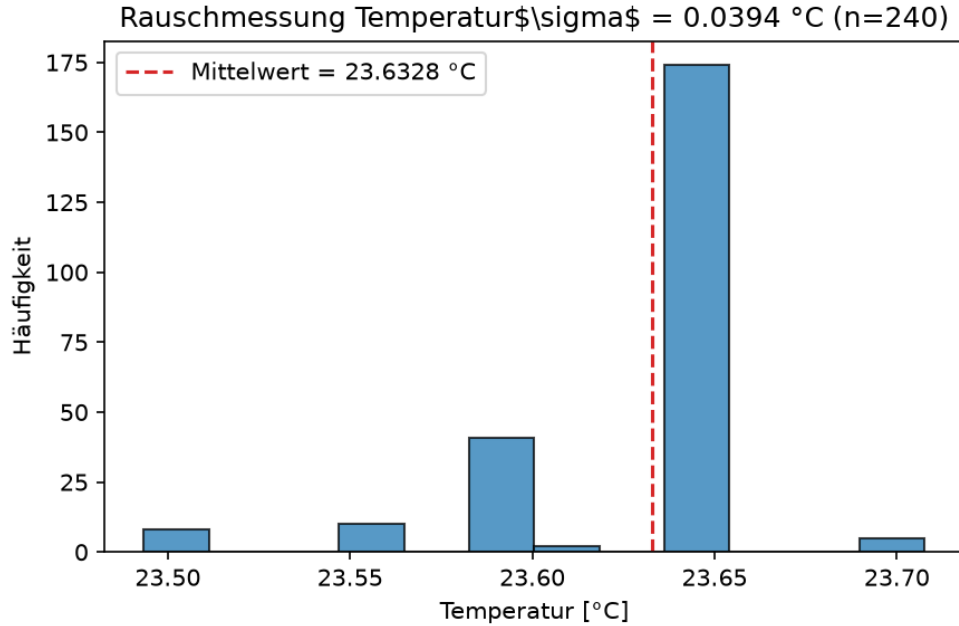
Abbildung 2: Rauschmessung der Temperatur vor dem Hauptversuch, mit Mittelwert und Standardabweichung.
